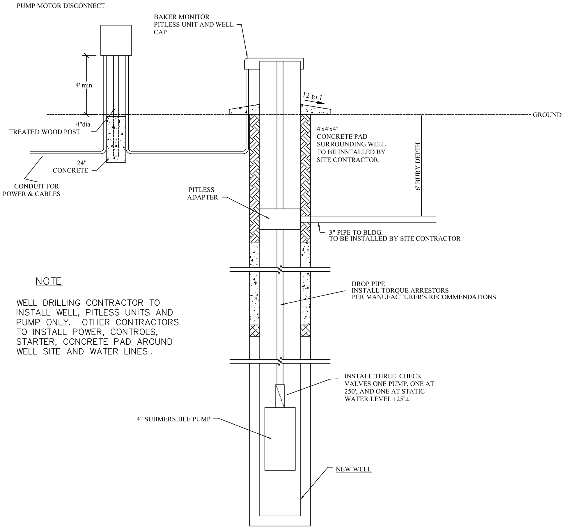
WELL DETAIL N.T.S.
